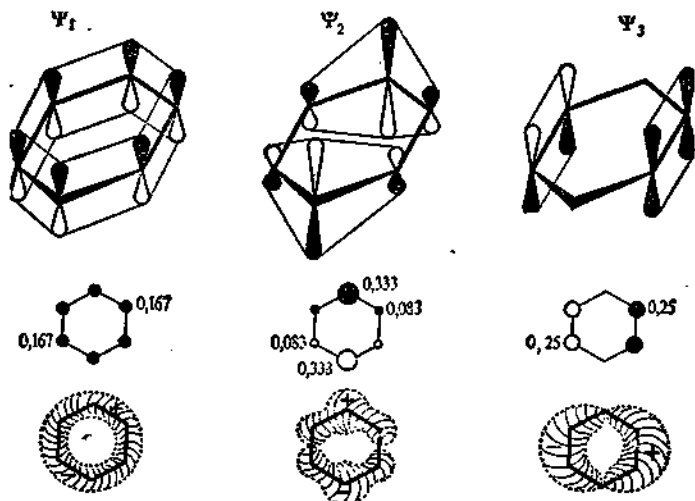
Рис. 68. Очертания заполненных МО бензола и значения одноэлектронной плотности c_{jr}^2
