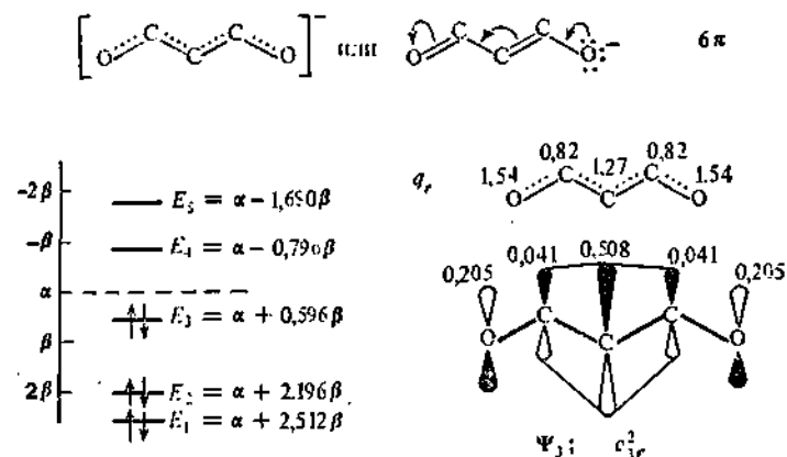
Рис. 98. Значения энергии МО, одноэлектронные плотности ВЗМО, плотность \pi -электронов транс -аниона \beta -дикетона
