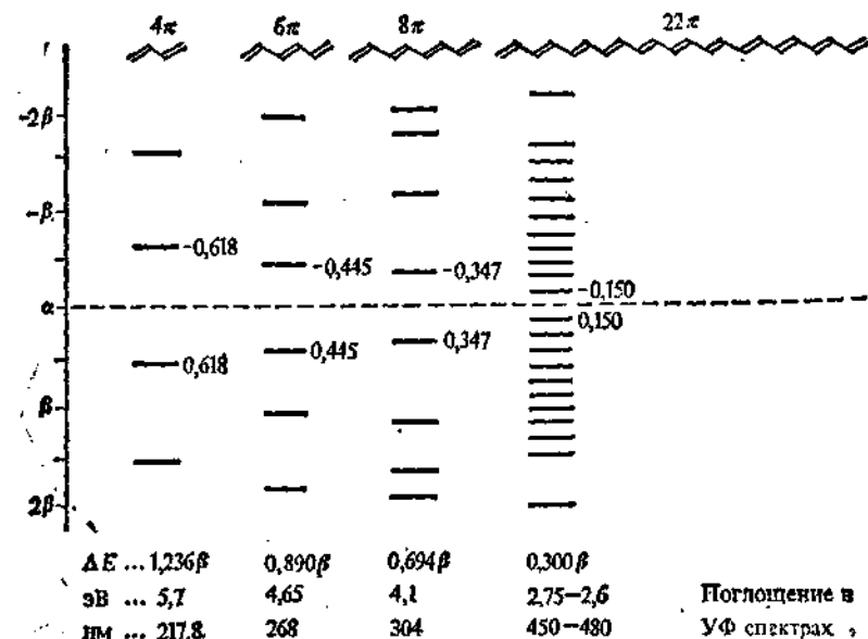
Рис. 61. Диаграммы уровней энергии некоторых полиенов и длинноволновые максимумы поглощения в электронных спектрах
