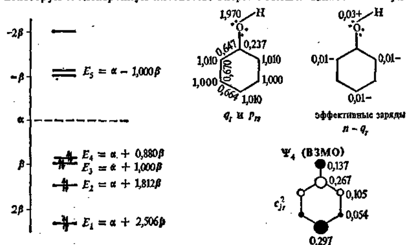
Рис. 86. Значения энергии МО, одноэлектронные плотности ВЗМО, плотность \pi -электронов, порядки \pi -связей и эффективные заряды \pi -электронной системы фенола
