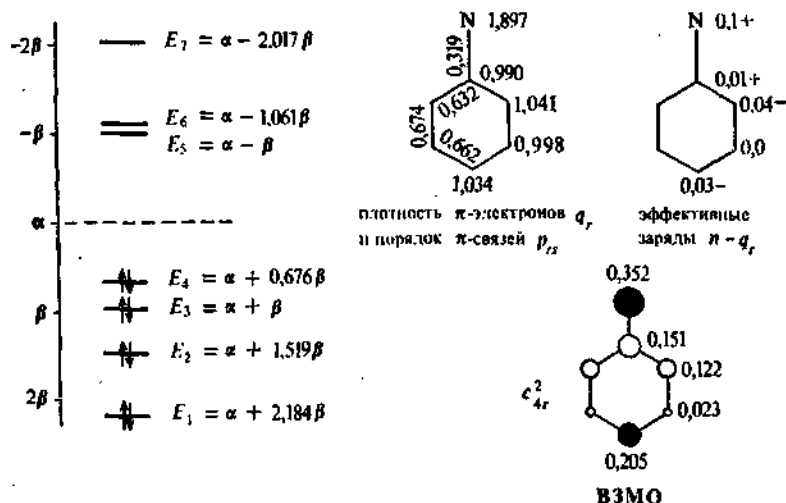
Рис. 94. Значения энергии МО, одноэлектронные плотности ВЗМО, плотность \pi -электронов, порядки \pi -связей и эффективные заряды \pi -электронной системы анилина
