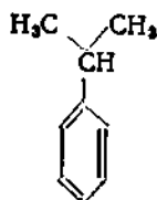
кумол (изопропил- бензол)
