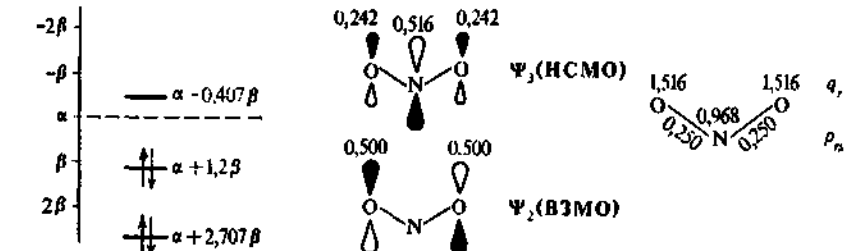
Рис. 90. Значения энергии МО, одноэлектронные плотности фронтальных орбиталей, плотность \pi -электронов и порядки \pi -связей нитрогруппы
