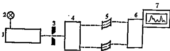
Рис. 29. Принципиальная схема двухлучевого прибора:
