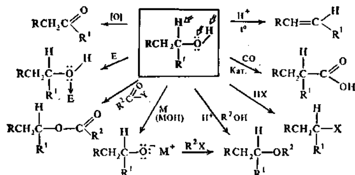
Реакции с сохранением атома кислорода в молекуле Реакции с отщеплением гидроксильной группы Рис. 84. Характерные реакции алканолов
