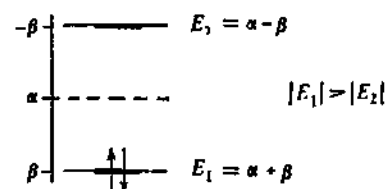
Рис. 52. Уровни энергии \pi -связи этилена и значения энергии
