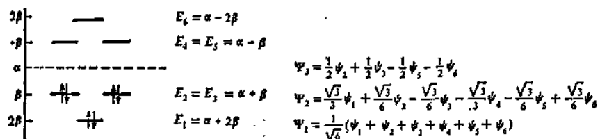
Рис. 67. Диаграмма энергетических уровней бензола и значения собственных векторов заполненных МО
