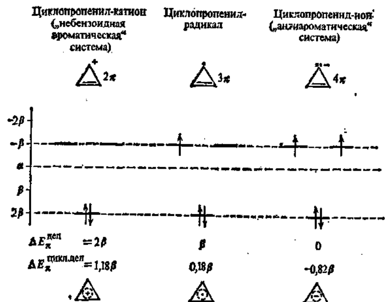
Рис. 75. Расположение МО и энергия делокализации и циклической делокализации трехчленных сопряженных систем
