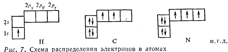
Рис. 7. Схема распределения электронов в атомах
