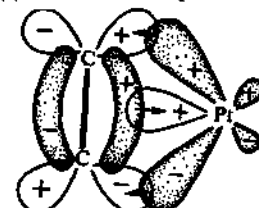
Рис. 82. Образование связи в π-комплексе алкен — металл (заполненные орбитали заштрихованы, незаполненные и разрыхляющие незаштрихованы)
