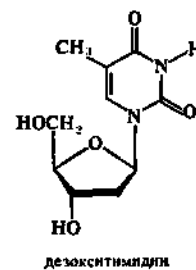
дезокситимидин
