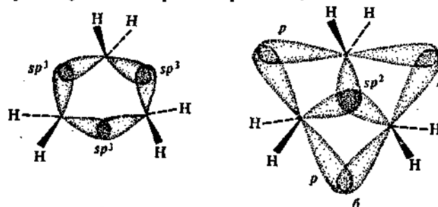
Рис. 66. Образование связей в молекуле циклопропана
