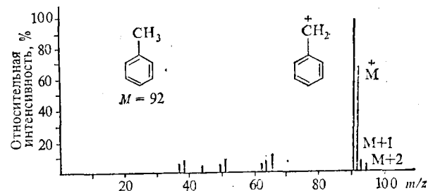
Рис. 46. Масс-спектр толуола
