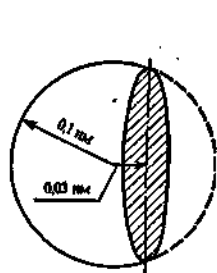
Рис. 21. Модель атома водорода
