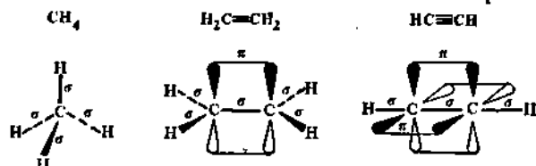
Рис. 15. Образование \sigma - и \pi -связей
