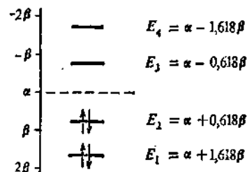
Рис. 59. Уровни энергии, значения энергии МО \pi -электронной системы молекулы бутадиена-1,3
