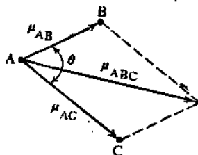
Рис. 19. Суммирование дипольных моментов связей:
