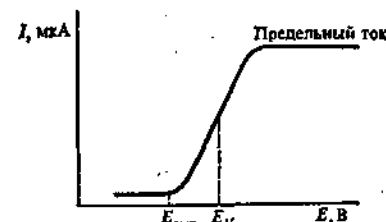
Рис. 27. Полярограмма
