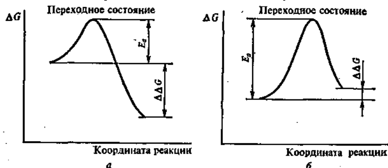
Рис. 47. Изменение свободной энергии в ходе реакции:
