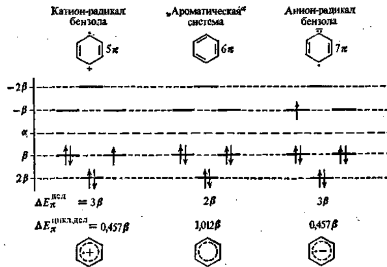
Рис. 78. Расположение МО и энергия делокализации и циклической делокализации шестичленных сопряженных систем
