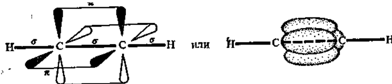
Рис. 62. Образование π-связей в молекуле ацетилена
