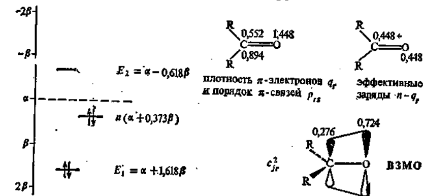
Рис. 97. Значения энергии МО, одноэлектронные плотности ВЗМО, плотность \pi -электронов, порядок \pi -связи и эффективные заряды карбонильной группы
