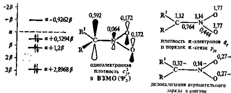
Рис. 91. Значения энергии МО, одноэлектронные плотности ВЗМО, плотность π-электронов, порядки π-связей и делокализация отрицательного заряда в нитронат-ионе
