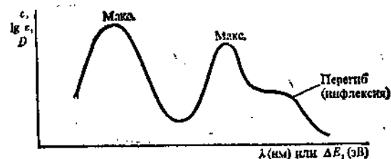
Рис. 30. Спектр поглощения
