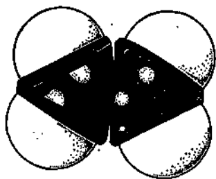
Рис. 24. Модель молекулы этилена
