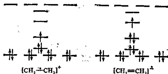
Рис. 18. Распределение электронов по орбиталам катион-радикала и анион-радикала этилена
