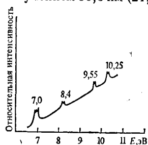
Рис. 45. Фотоэлектронный спектр тетрацена
