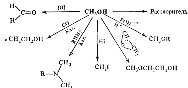
Рис. 85. Схема использования метанола
