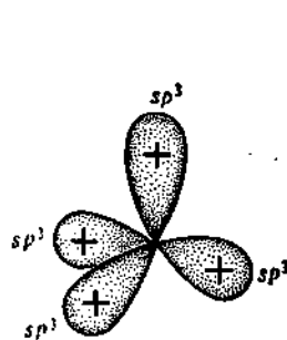
Рис. 12. sp^3 -Гибридизация орбиталей
