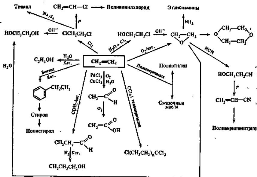
Рис. 56. Применение этилена
