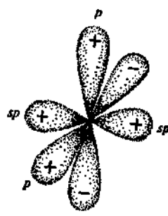
Рис. 14. sp -Гибридизация орбиталей
