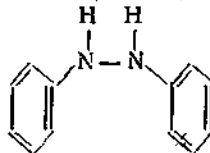
N,N' -дифенилгидразин, гидразобензол
