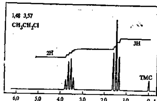
Рис. 39. Спектр ПМР этилхлорида в растворе \text{CDCl}_3
