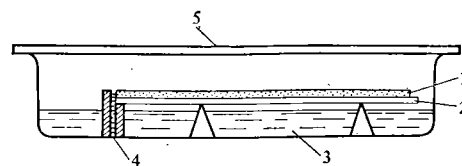
Рис. 2. Установка для тонкослойной хроматографии: 1 — сорбент; 2 — пластинка; 3 — элюент; 4 — капиллярная щель; 5 — крышка
