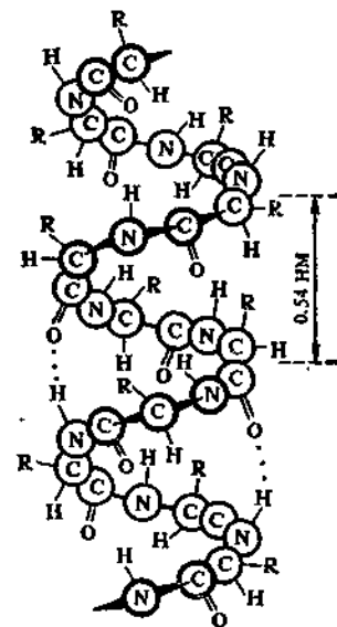
Рис. 99. Правая \alpha -спираль полипептида
