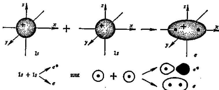
Рис. 9. Образование \sigma -связи ( \sigma^* — разрыхляющая \sigma -орбиталь)
