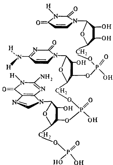
Рис. 101. Тринуклеотид из гуанина, цитозина и урацила, pGpCpU
