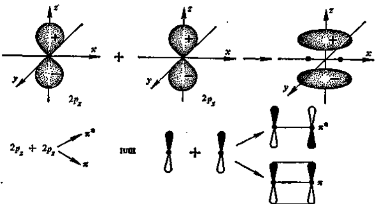
Рис. 10. Образование \pi -связи ( \pi^* — разрыхляющая \pi -орбиталь)
