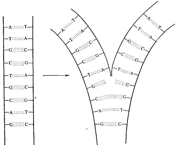
Рис. 104. Схема репликации двуцепочечного комплекса ДНК (двойной спирали). Упрощенно обе цепи нарисованы растянутыми
