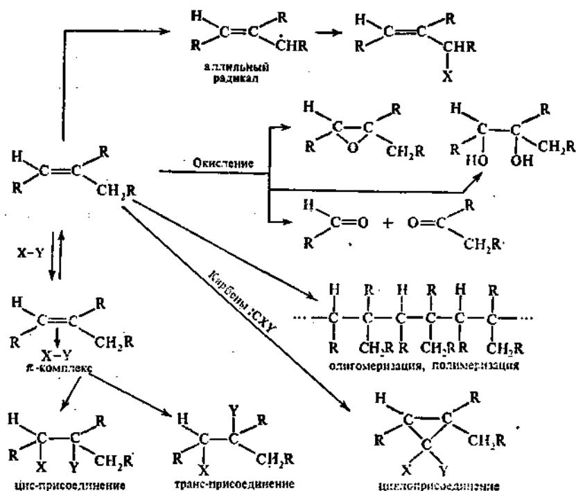
Рис. 51. Схема превращений алкенов
