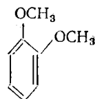
1,2-диметоксibenзол, вератрол (диметиловый эфир пирокатехина)
