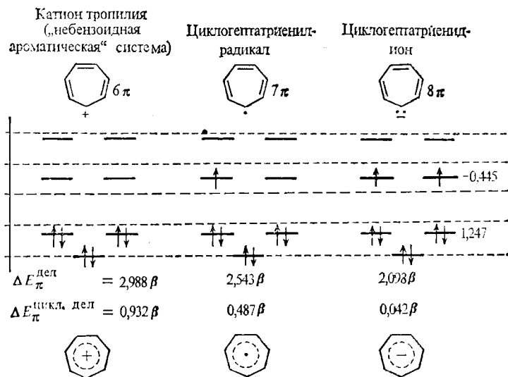
Рис. 79. Расположение МО и энергия делокализации и циклической делокализации семичленных сопряженных систем
