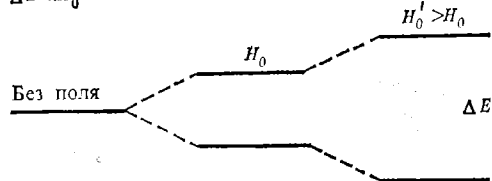
Рис. 35. Расщепление энергетических уровней спинового магнитного момента в магнитном поле
