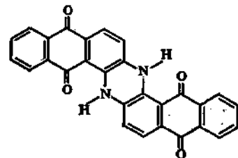
индантрон (кубовый синий O)
