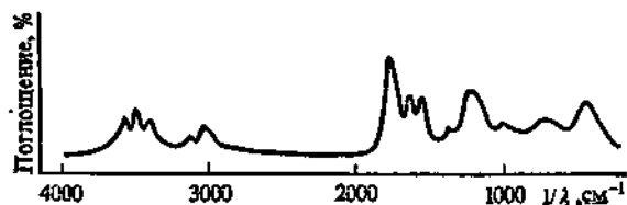
Рис. 33. Изображение инфракрасного спектра поглощения
