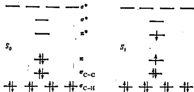
Рис. 17. Возбуждение молекулы этилена ( \pi \rightarrow \pi^* -переход)
