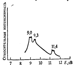
Рис. 44. Фотоэлектронный спектр толуола
