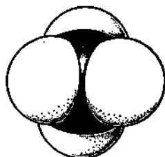
Рис. 23. Модель молекулы метана
