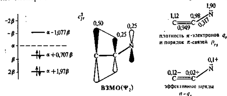
Рис. 93. Значения энергии МО, одноэлектронные плотности ВЗМО, плотность \pi -электронов, порядки \pi -связей и эффективные заряды \pi -электронной системы енамина
