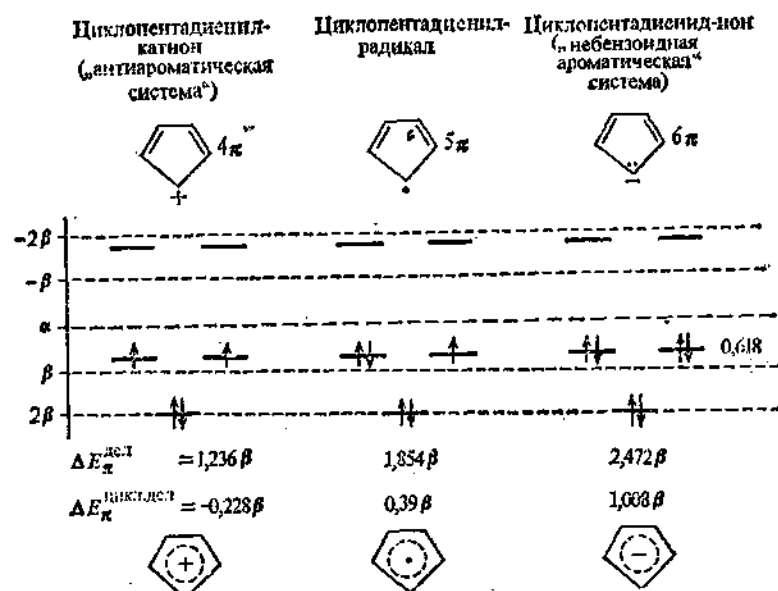
Рис. 77. Расположение МО и энергия делокализации и циклической делокализации пятичленных сопряженных систем
