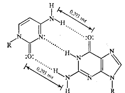
Рис. 103. Комплементарные пары тимин-аденин с двумя водородными связями и цитозин-гуанин с тремя водородными связями
