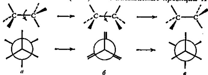
Рис. 48. Вращение в молекуле этана:
