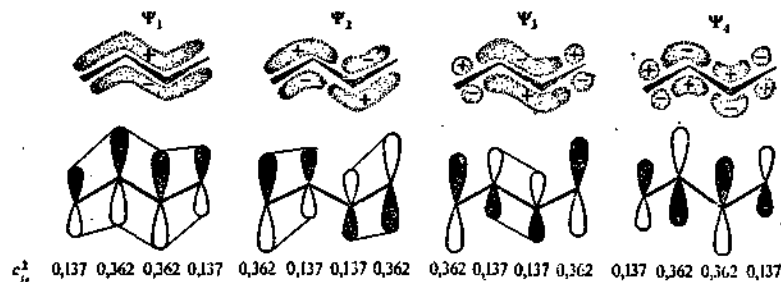
Рис. 60. Очертания МО молекулы бутадиена-1,3
