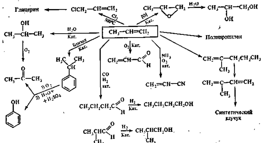
Рис. 57. Применение пропена
