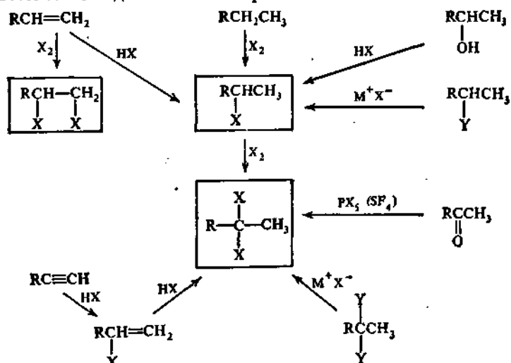
Рис. 80. Генетическая связь между углеводородами, их галогенпроизводными и кислородсодержащими соединениями
