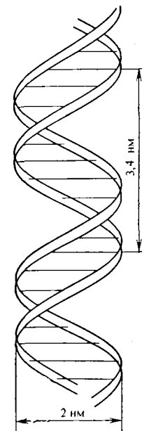
Рис. 102. Схема двойной спирали ДНК
