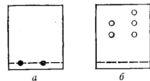
Рис. 3. Тонкослойная хроматограмма: а — до элюации; б — после элюации
