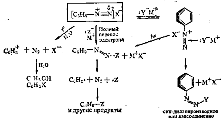
Схема 1. Превращение солей диазона
