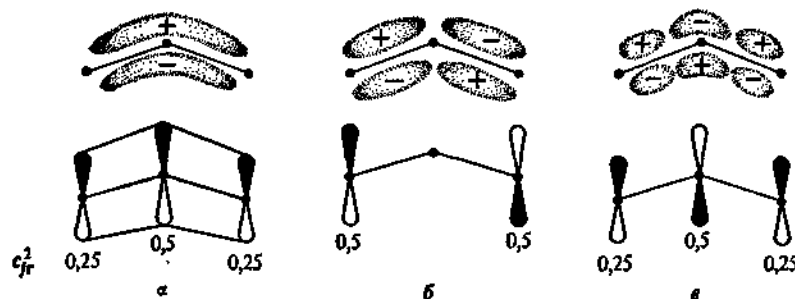
Рис. 55. Очертания МО аллильного радикала:
