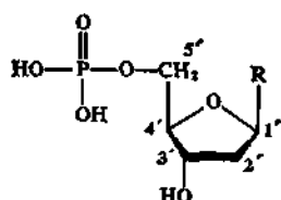
дезоксирибонуклеотиды
