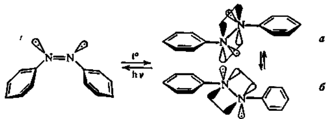
Рис. 96. Пространственная изомерия азоаренов
