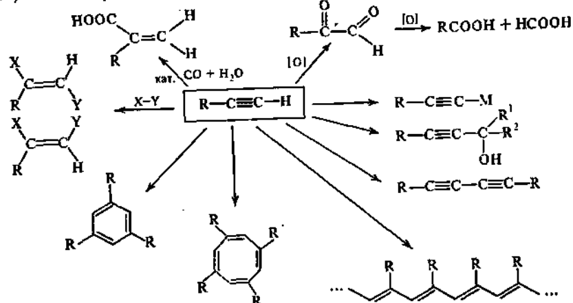
Рис. 63. Характерные реакции алкинов
