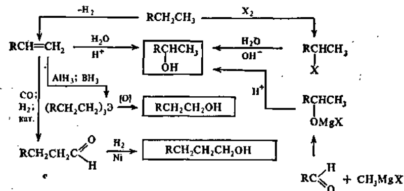
Рис. 83. Генетическая связь между алканолами, алканами, алкенами и карбонильными соединениями
