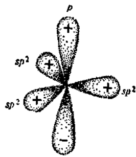
Рис. 13. sp^2 -Гибридизация орбиталей
