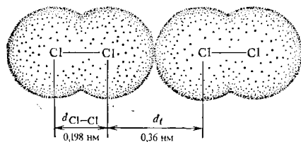
Рис. 20. Радиус эффективного действия молекулы хлора
