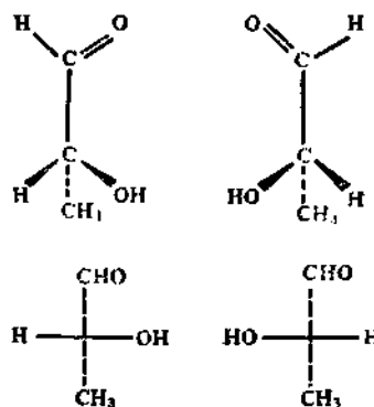
R - \alpha -гидроксипропионовый альдегид S - \alpha -гидроксипропионовый альдегид
