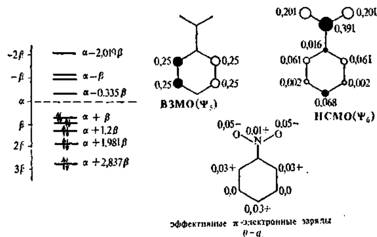
Рис. 92. Значения энергии МО, одноэлектронные плотности фронтальных орбиталей, эффективные заряды π-электронной системы нитробензола
