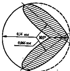
Рис. 22. Модель атома кислорода
