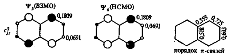
Рис. 74. Одноэлектронная плотность во фронтальных орбиталях нафталина и порядок \pi -связей
