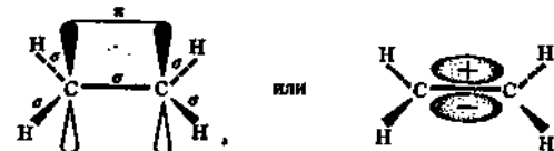
Рис. 50. Типы связей в молекуле этилена
