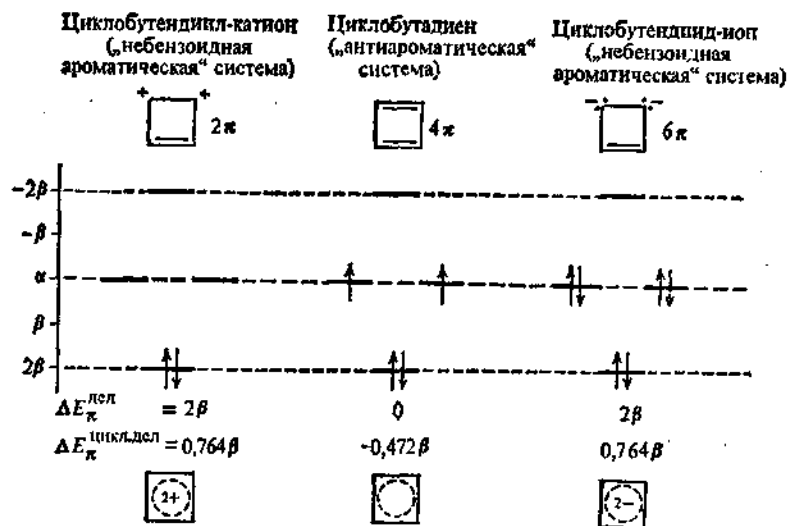
Рис. 76. Расположение МО и энергия делокализации и циклической делокализации четырехчленных сопряженных систем
