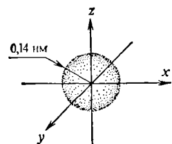
Рис. 5. s -Орбиталь
