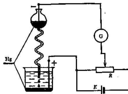
Рис. 26. Принципиальная схема полярографа
