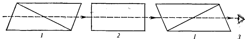
Рис. 43. Схематичное изображение поляриметра: 1 — призмы Николя; 2 — трубка с веществом; 3 — глаз наблюдателя
