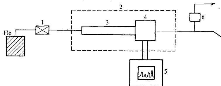
Рис. 4. Принципиальная схема газового хроматографа: 1 — регулятор потока газа-носителя; 2 — термостат; 3 — адсорбционная колонка; 4 — детектор; 5 — самописец; 6 — установка для улавливания фракций
